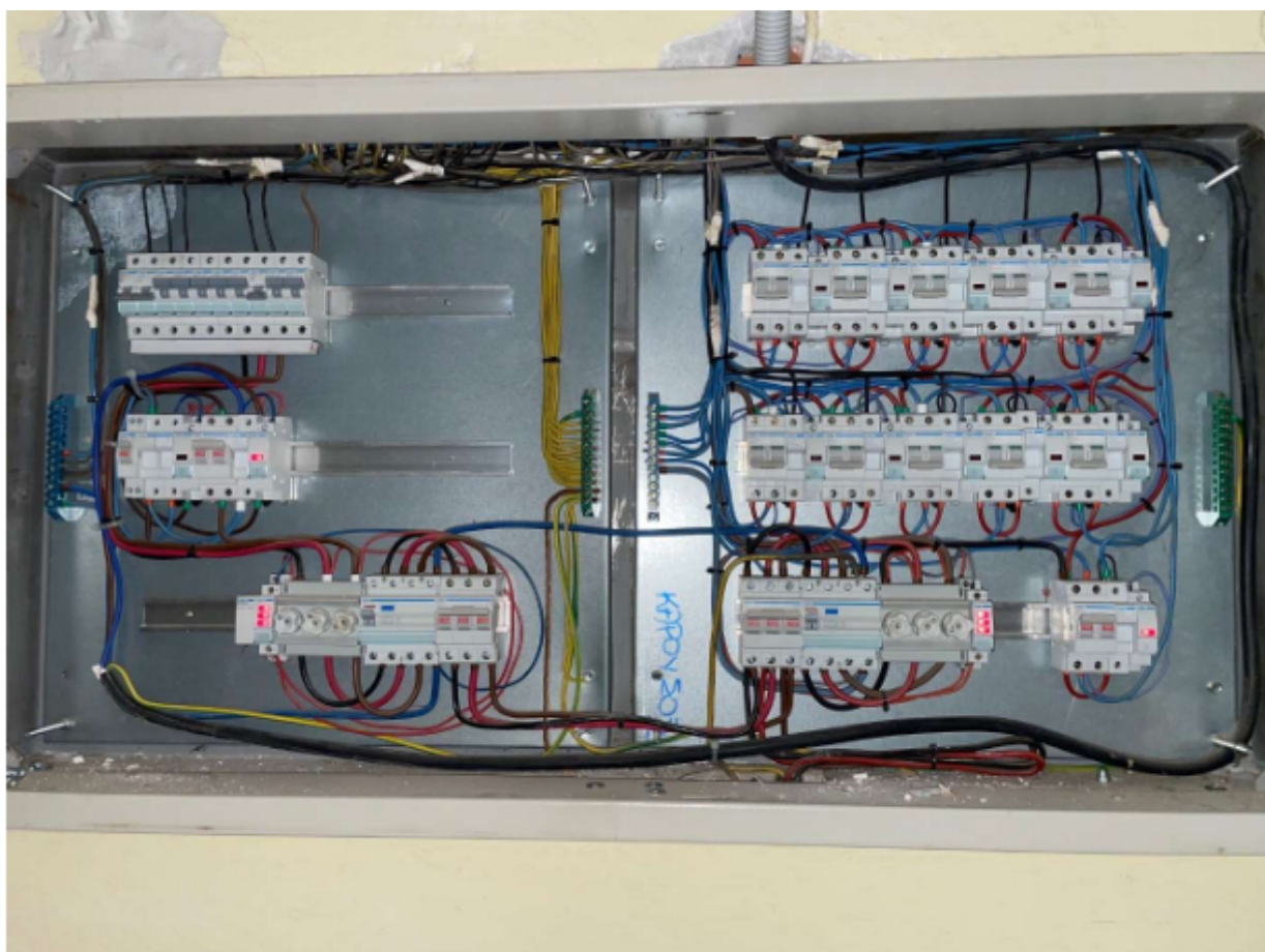
Εικόνα 16(Ηλ.Πίνακας διαδρόμου Α ορόφου προς Αυλή)
