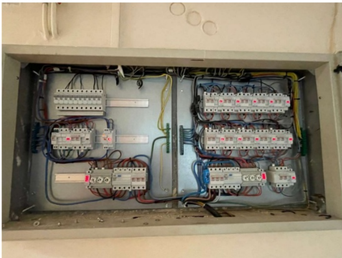
Εικόνα 21(Ηλ.πίνακας Β όροφος προς ΚΑΠΗ)
