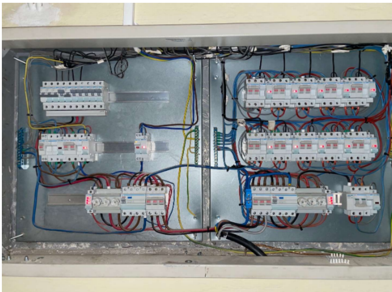
Εικόνα 15(Ηλ.Πίνακας διαδρόμου Α ορόφου προς ΚΑΠΗ)
